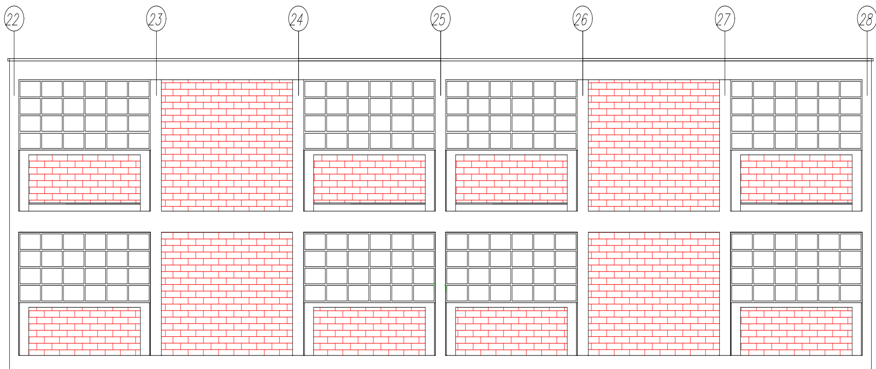
ELEVACION EXTERIOR INCLUYENDO MUROS DE ALBAÑILERIA CERRANDO 2 PAÑOS COMPLETOS
